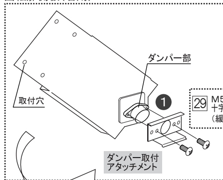
回転扉側板(右用)
